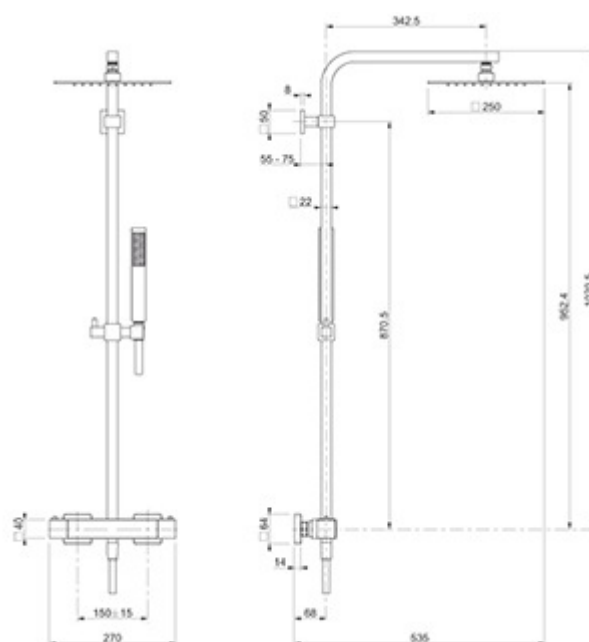
Schéma technique
