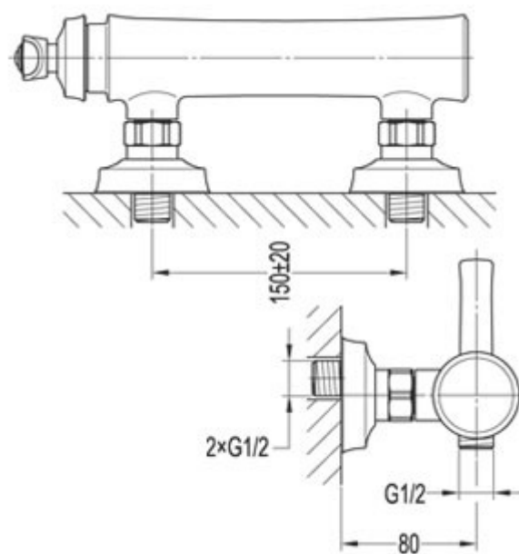
Schéma technique
