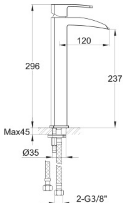
Schéma technique
