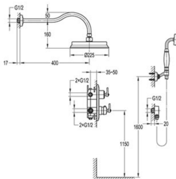
Schéma technique
