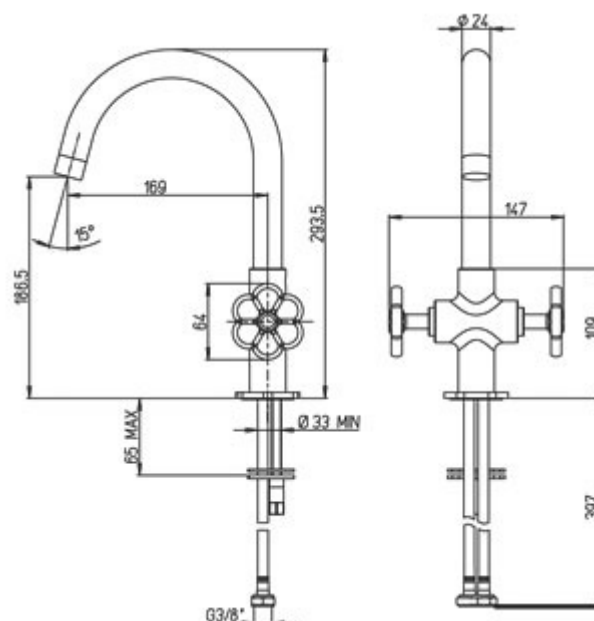
Schéma technique
