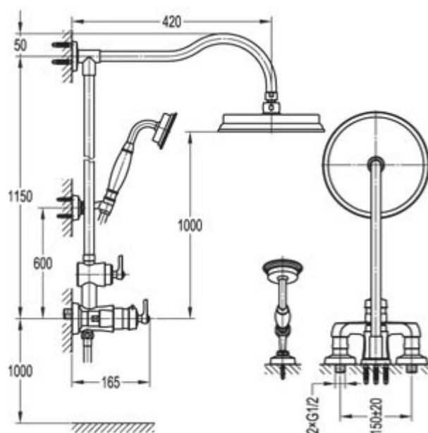
Schéma technique
